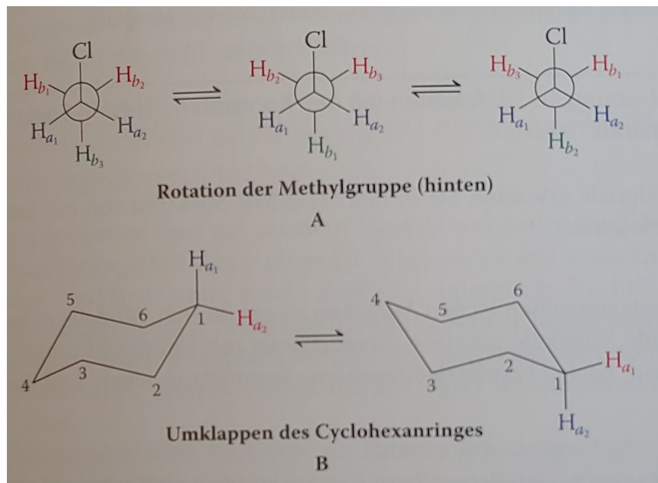
Figure 12: Symmetrieoperationen am Beispiel Chlorethan (A) und Cyclohexan (B). Bei Chlorethan kann eine Spiegelachse vertikal von Chlor (Cl) zum unteren Wasserstoff (grün) gezogen werden. Ebenso ist eine Rotationsachse zwischen den beiden Kohlenstoffen (Kreismitte) möglich. In Cyclohexan steht ein Wasserstoff orthogonal (axial) und einer waagrecht (äquatorial) zum 6-Ring. Durch ein ändern der Sesselkonfiguration, können beide aber ineinander überführt werden [4].
