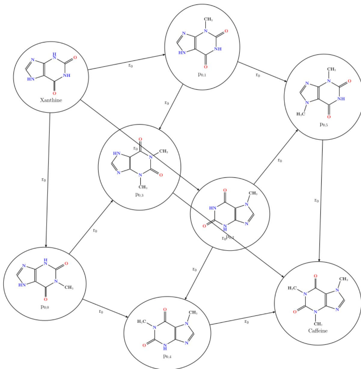
Abbildung 4.5: Darstellung aller Synthesepfade von Koffein aus Xanthin in dem Grap- transformationstool. Die Graphen p_{0,0} bis p_{0,5} stellen dabei die Zwischenprodukte 1- Methylxanthin, 3-Methylxanthin, 7-Methylxanthin, 1,3-Dimethylxanthin oder Theophyl- line, 1,7-Dimethylxanthin oder Paraxanthin und 3,7-Dimethylxanthin oder Theobromin dar.
