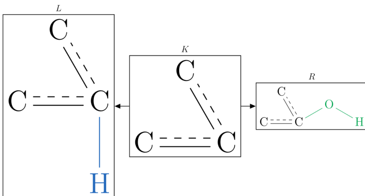
Abbildung 4.7: Darstellung der Regel zum Hydroxylieren des Phenylrests in dem Graphtransformationstool.
