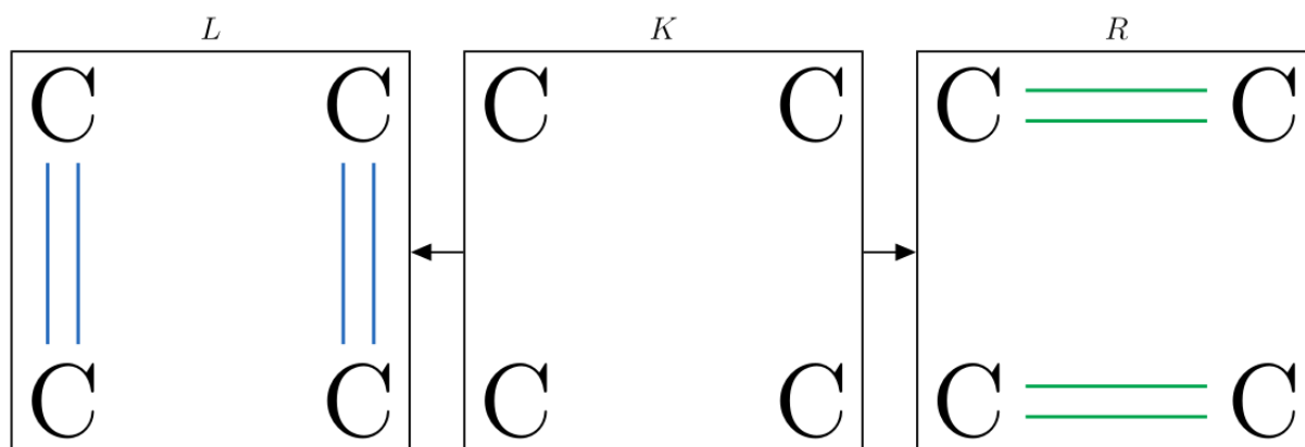
Abbildung 4.13: Olefin Metathese in dem Graptransformationstool.
