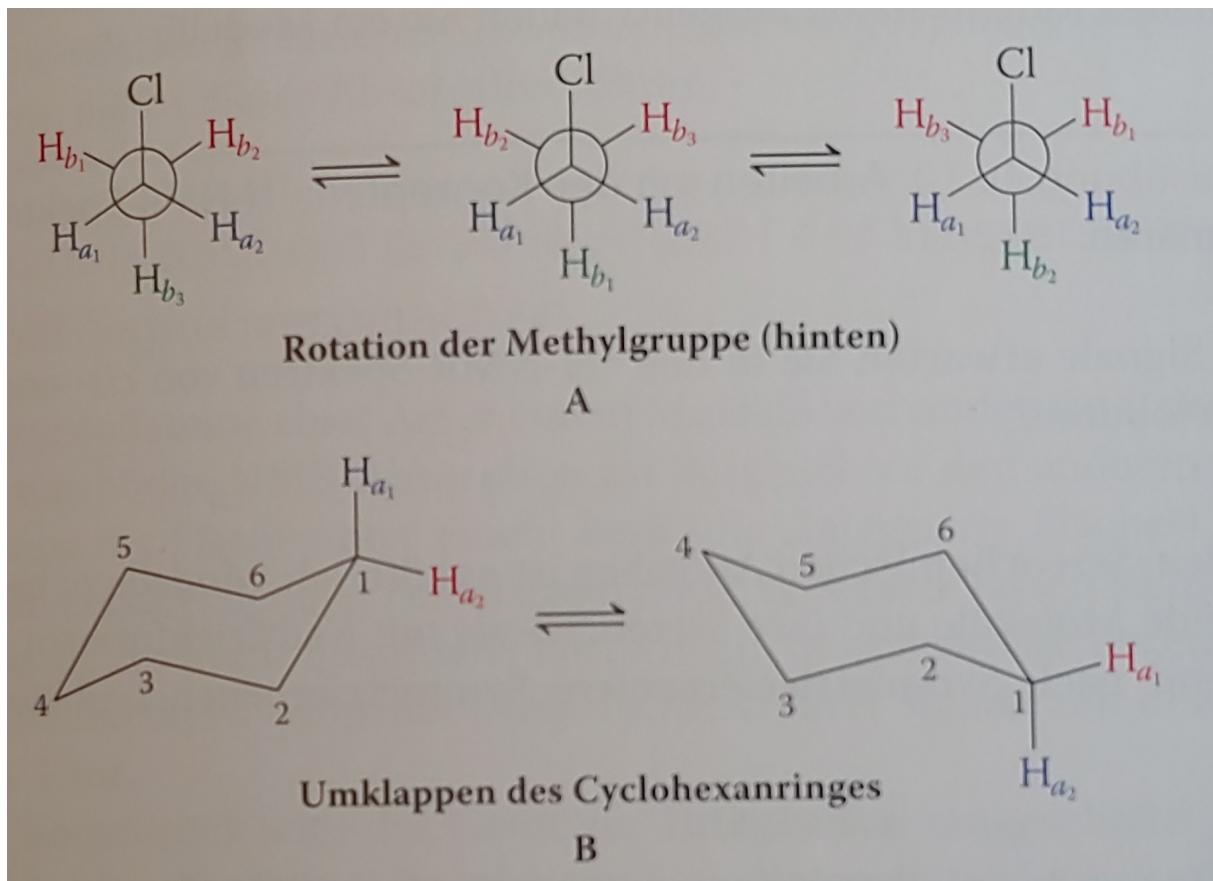
Abbildung 2.12: Symmetrioperationen am Beispiel Chlorethan (A) und Cyclohexan (B). Bei Chlorethan kann eine Spiegelachse vertikal von Chlor (Cl) zum unteren Wasserstoff (grün) gezogen werden. Ebenso ist eine Rotationsachse zwischen den beiden Kohlenstoffen (Kreismitte) möglich. In Cyclohexan steht ein Wasserstoff orthogonal (axial) und einer waagrecht (äquatorial) zum 6-Ring. Durch ein ändern der Sesselkonfiguration, können beide aber ineinander überführt werden [4].
