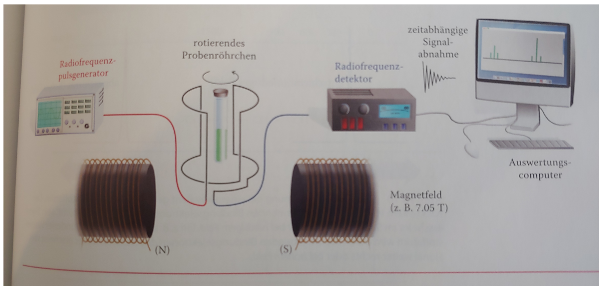
Abbildung 2.11: Schematischer Aufbau eines NMR-Spektrometers [4].
