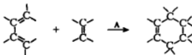
Abbildung 4.11: Die Diels Alder Reaktion [43].
