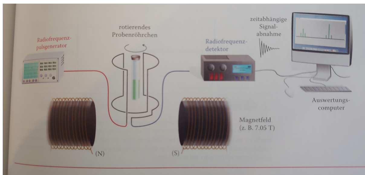
Abbildung 2.11: Schematischer Aufbau eines NMR-Spektrometers [5].
