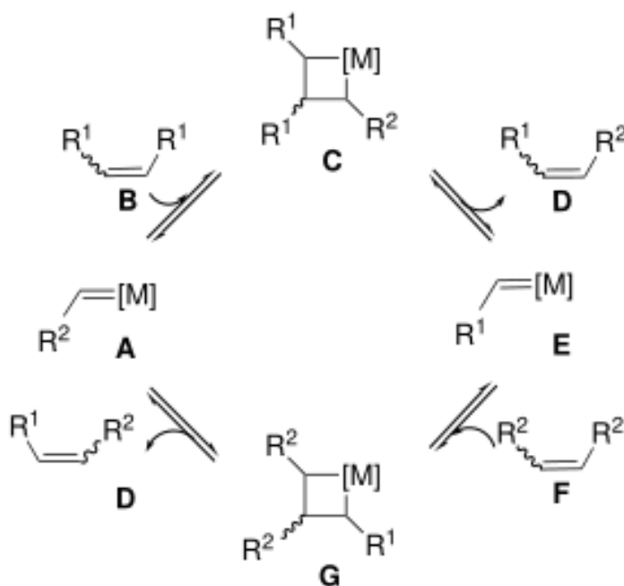
Abbildung 4.10: Katalysezyklus der Olefinmetathese [42].
