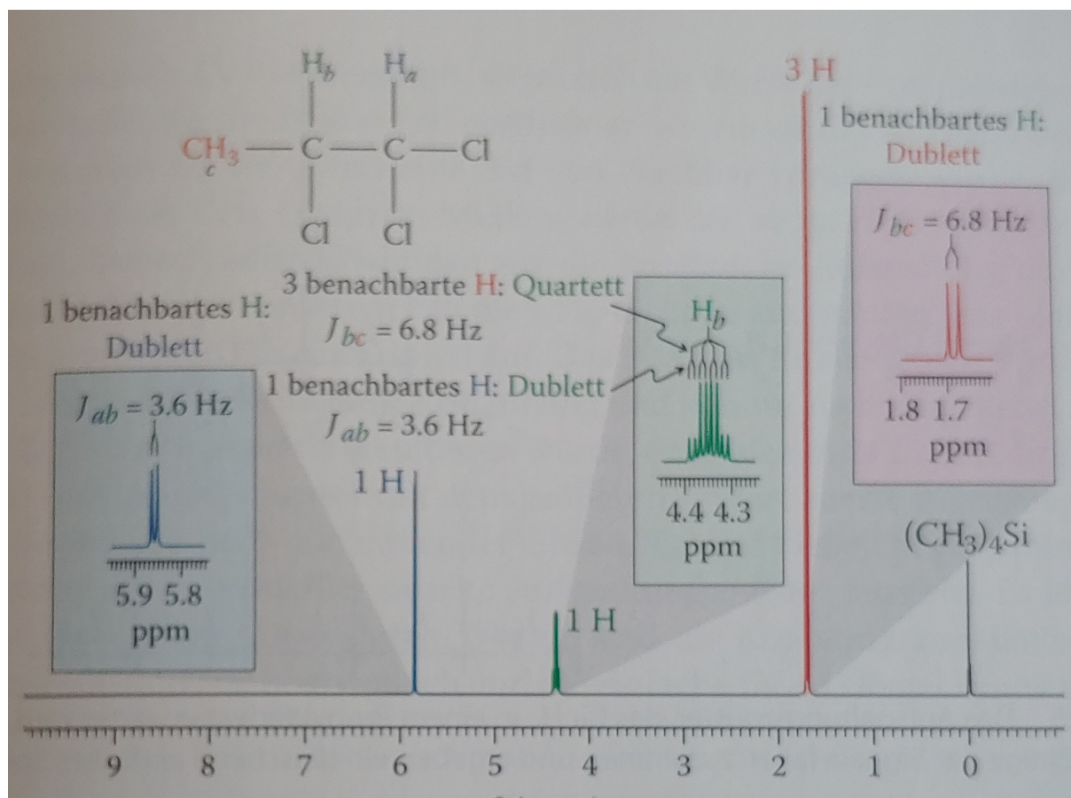
Abbildung 2.13: ^1\text{H} -NMR von 1,1,2-Trichlorpropan. Der Methylwasserstoff ( H_c rot) hat ein Dublett bei 1.68 ppm mit Intensität 3, der zentrale Wasserstoff ( H_b grün) hat bei 4.35 ein Dublett in Quartett mit Signalstärke 1 und der Endwasserstoff ( H_a blau) erzeugt ein Dublett bei 5.96 ppm mit Signalstärke 1 [3].
