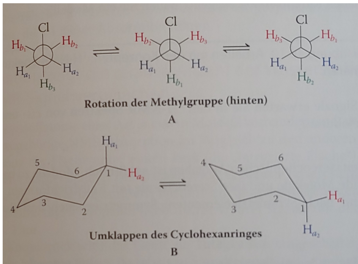
Abbildung 2.12: Symmetrieoperationen am Beispiel Chlorethan (A) und Cyclohexan (B). Bei Chlorethan kann eine Spiegelachse vertikal von Chlor (Cl) zum unteren Wasserstoff (grün) gezogen werden. Ebenso ist eine Rotationsachse zwischen den beiden Kohlenstoffen (Kreismitte) möglich. In Cyclohexan steht ein Wasserstoff orthogonal (axial) und einer waagrecht (äquatorial) zum 6-Ring. Durch ein ändern der Sesselkonfiguration, können beide aber ineinander überführt werden [3].
